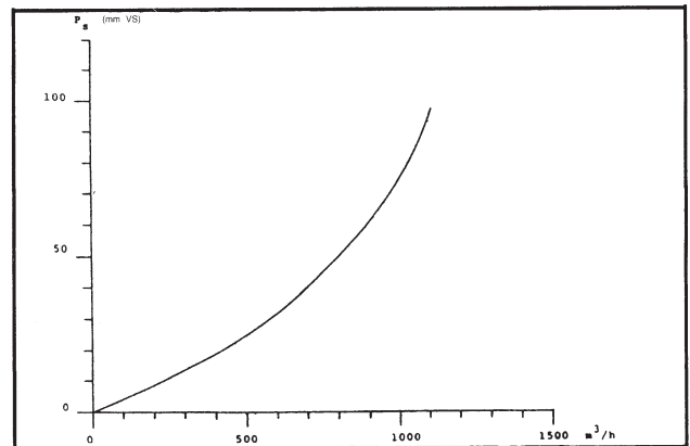
TRYKFALDSDIAGRAM 4,5 - 6 M ARM
