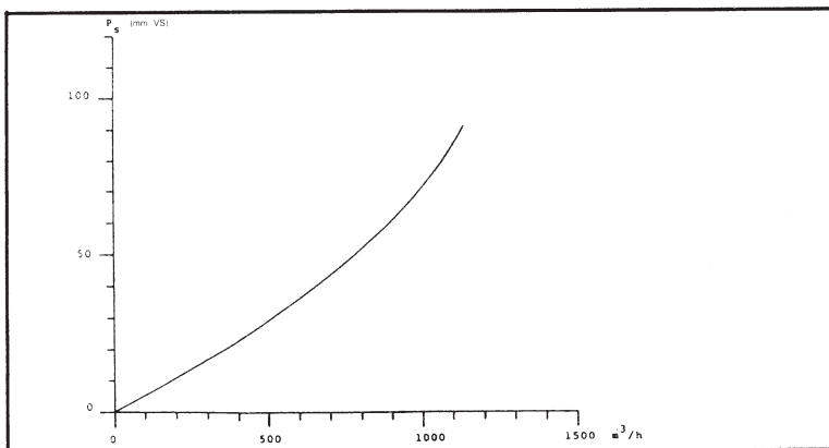
TRYKFALDSDIAGRAM 2 - 3 - 4 M ARM
